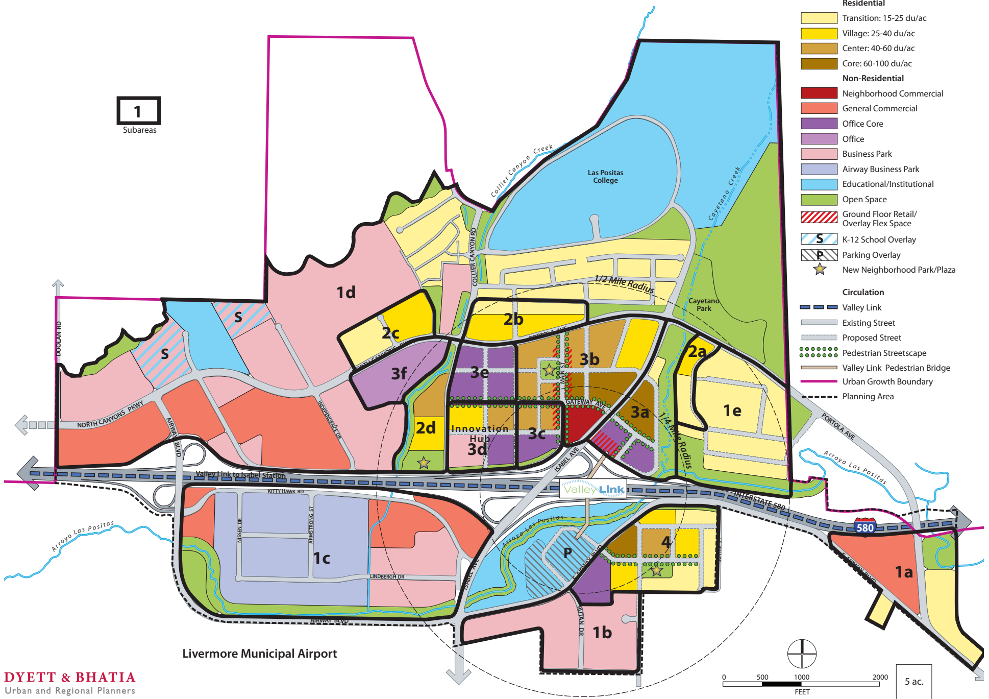
FIGURE 2-3: SUBAREA DIAGRAM
